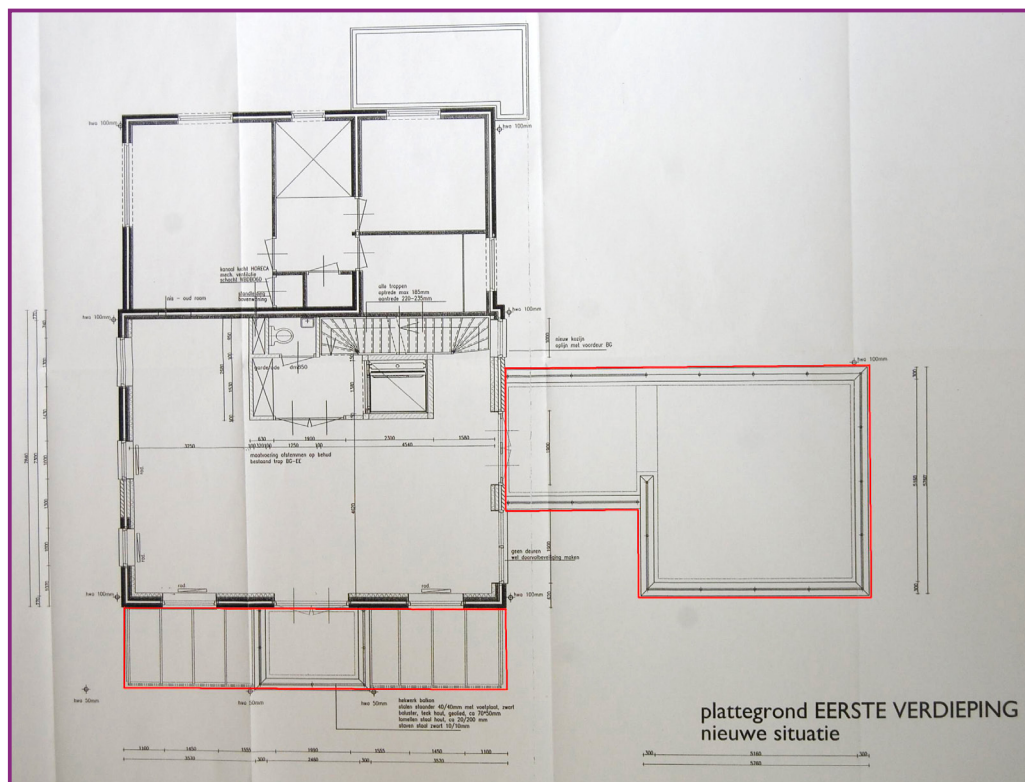
Afbeelding 2. Plattegrond van de geplande aanbouw in rood kader op een tekening van de bestaande bebouwing in zwart (noord is onder).
